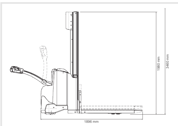
Dimensões principais (a)
